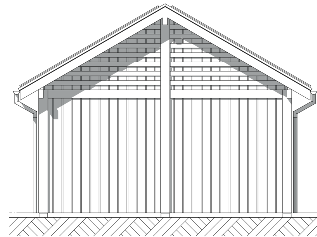
Linkergevel
