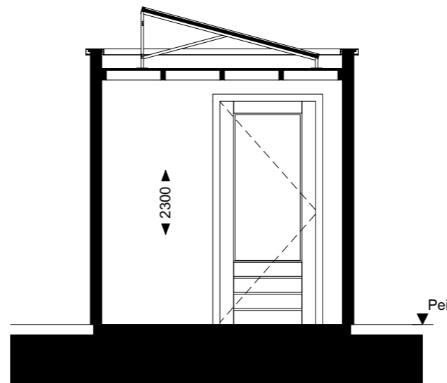
Doorsnede
