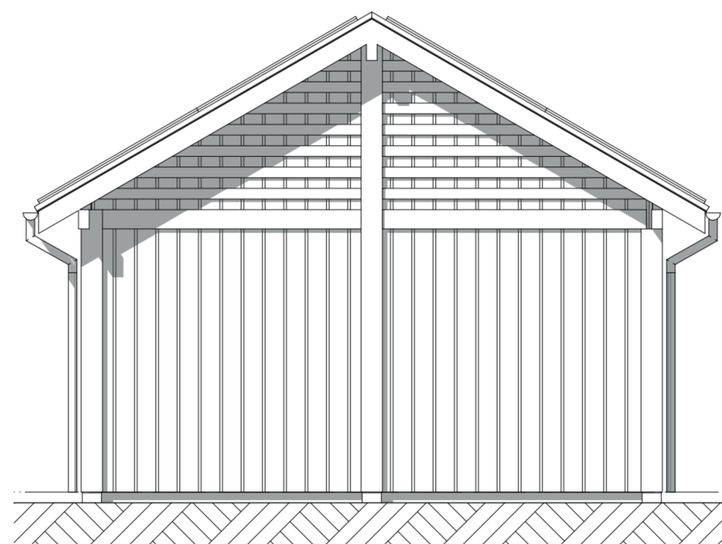
Linkergevel
