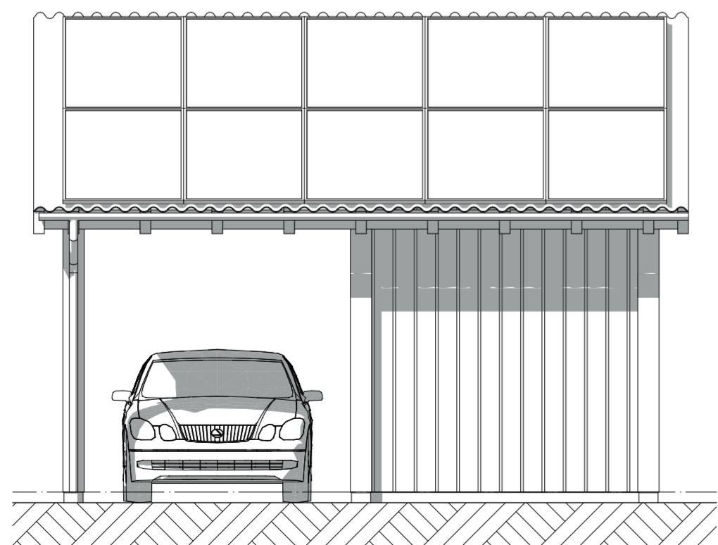
Achtergevel
