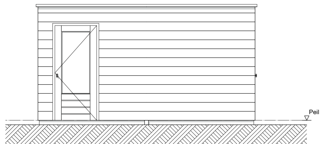
Achtergevel
