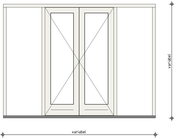
optie openslaande deuren met zijlichten achtergevel woningtypen: A, B, C, D en F
