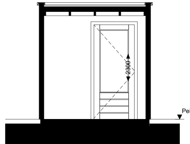
Doorsnede A-A dubbel
