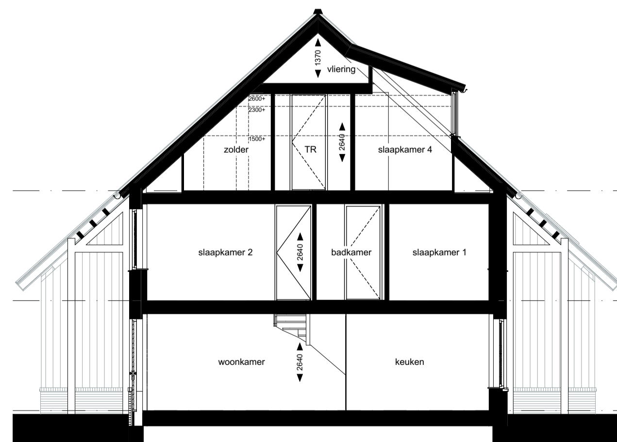
Doorsnede bnr. 135 1:100
