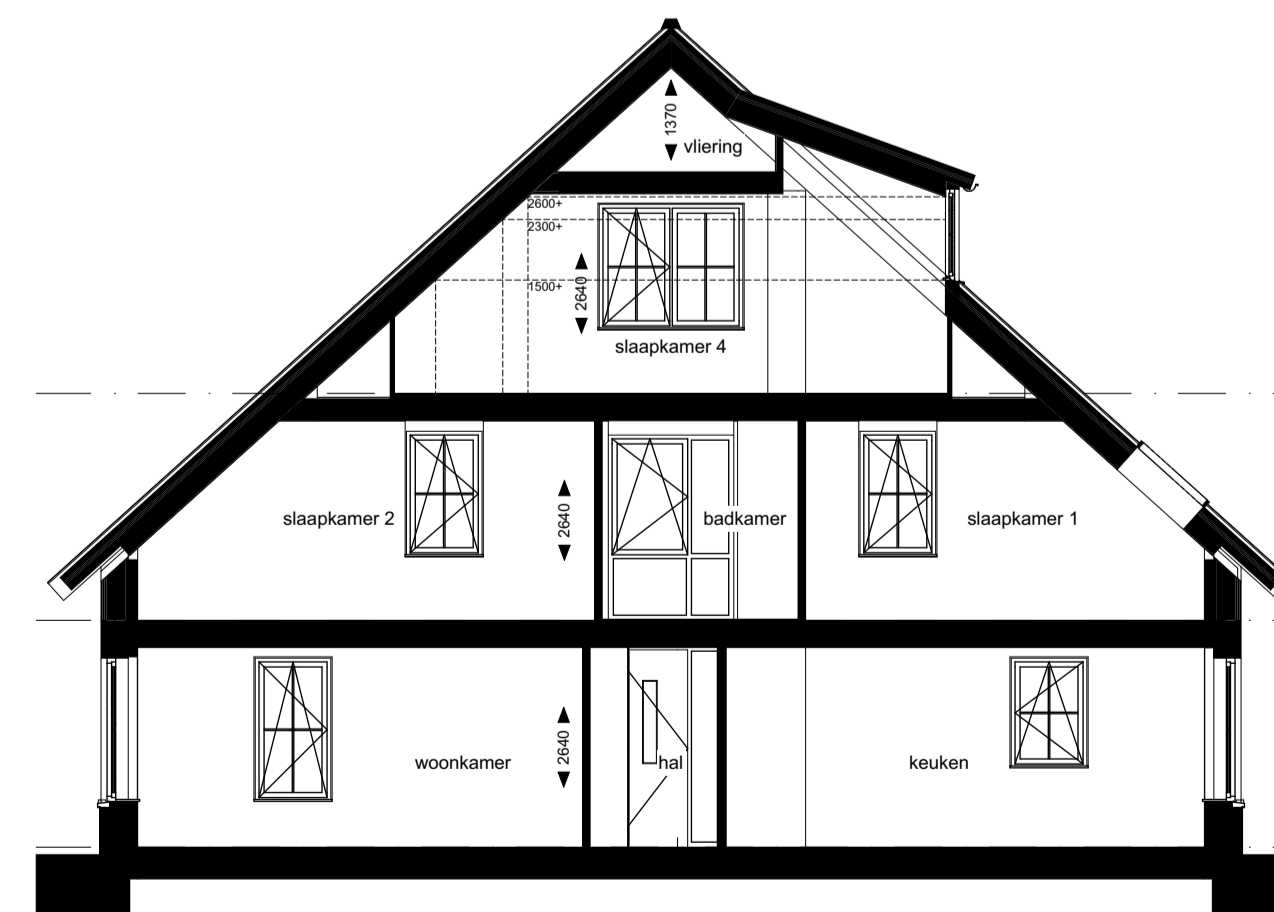
Doorsnede bnr. 136 1:100
