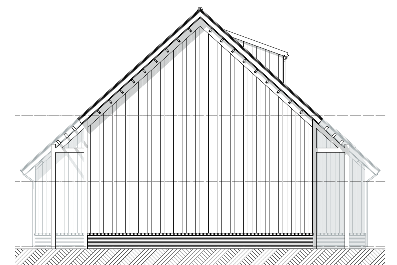
Bnr. 134 Linkergevel 1:100
