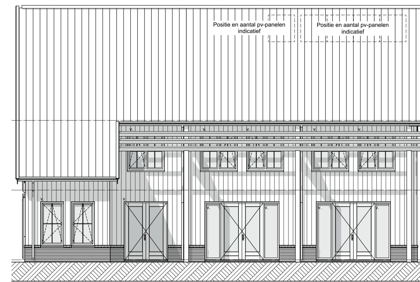
Bnr. 136 Bnr. 135 Bnr. 134 Achtergevel 1:100
