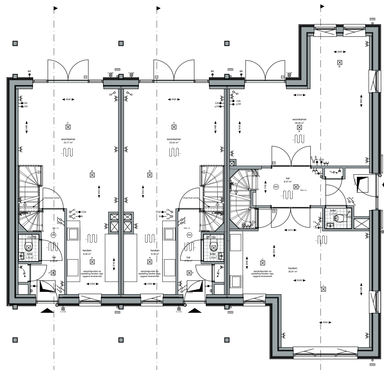
Bnr. 134 Bnr. 135 Bnr. 136 00 Begane grond 1:100
