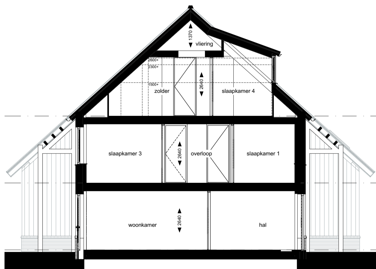
Doorsnede bnr. 134 1:100
