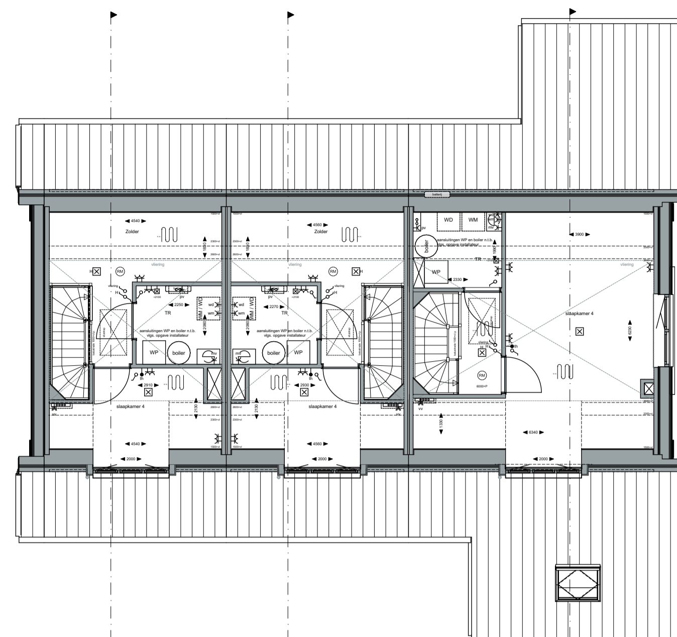
Bnr. 134 Bnr. 135 Bnr. 136 02 2e verdieping 1:100
