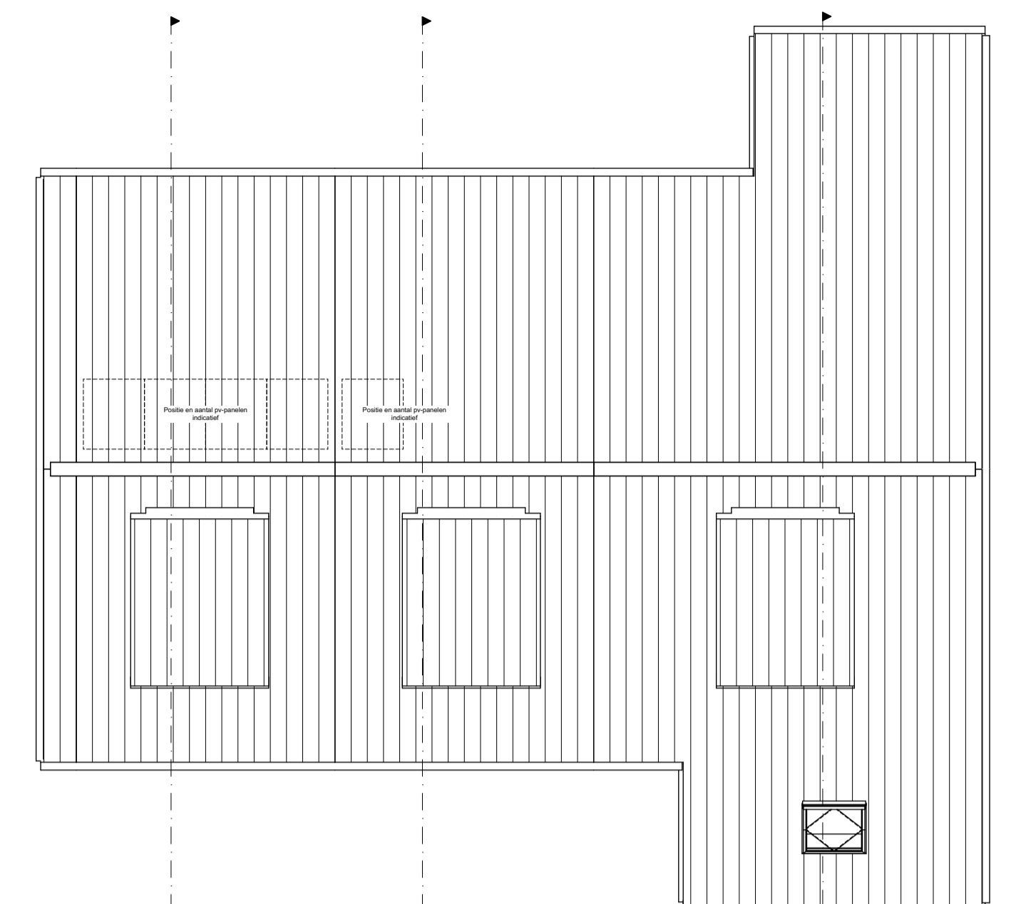
Bnr. 134 Bnr. 135 Bnr. 136 03 dakaanzicht 1:100
