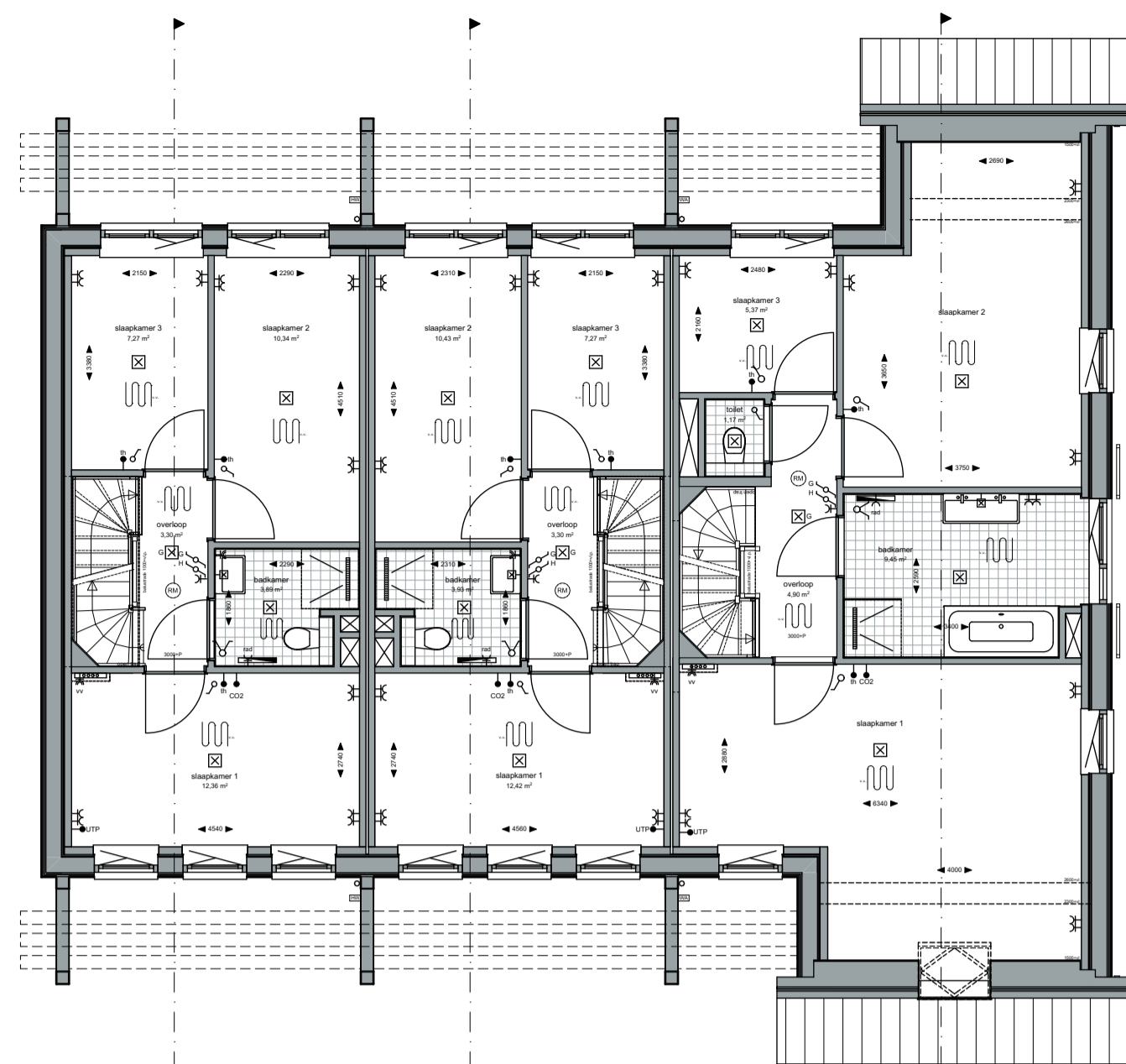
Bnr. 134 Bnr. 135 Bnr. 136 01 1e verdieping 1:100
