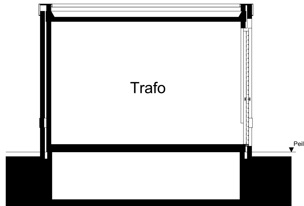
Doorsnede A-A
